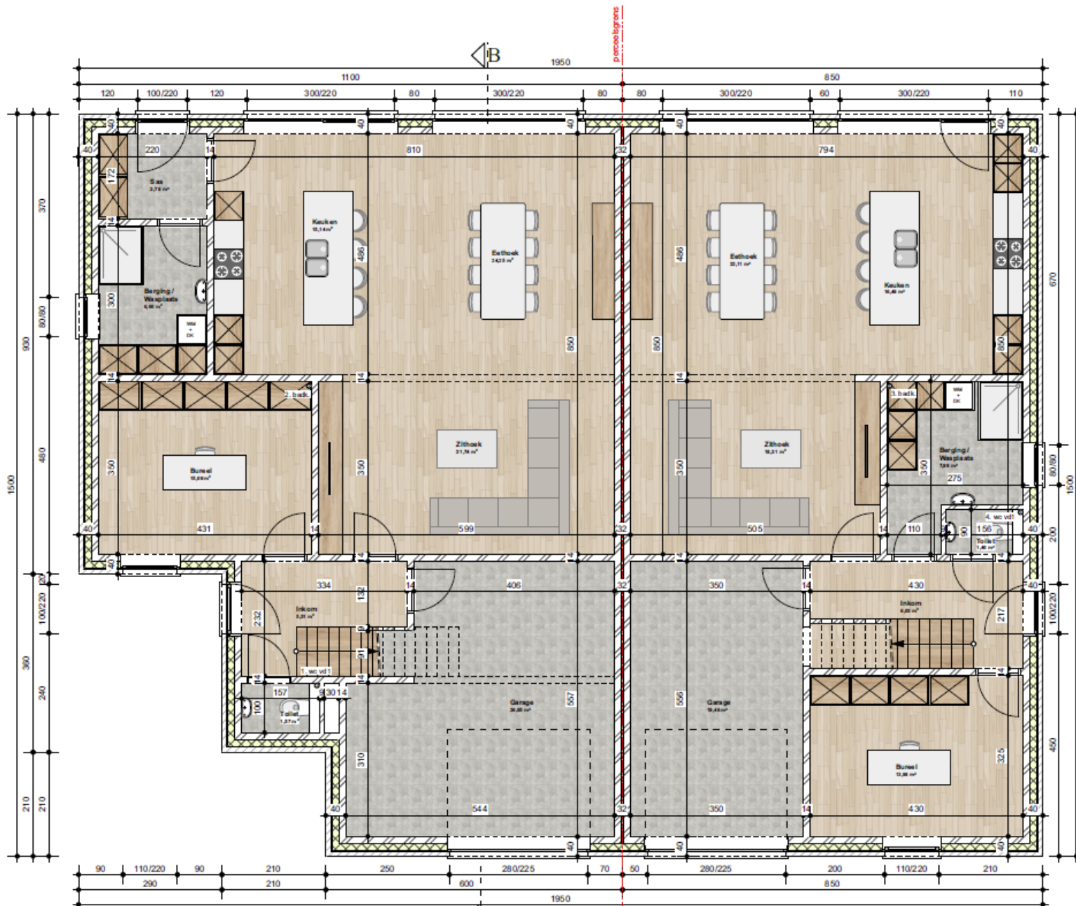
Grondplan gelijkvloers schaal 1/75
