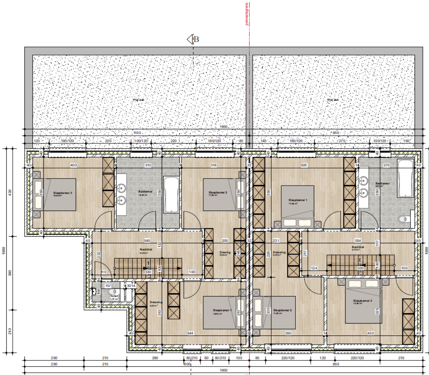
Grondplan verdieping schaal 1/75
